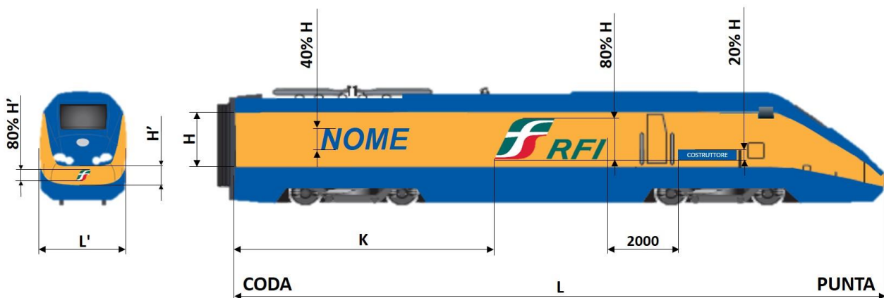
Figura 7 – Esempio iscrizioni locomotiva a singola cabina fiancata B
