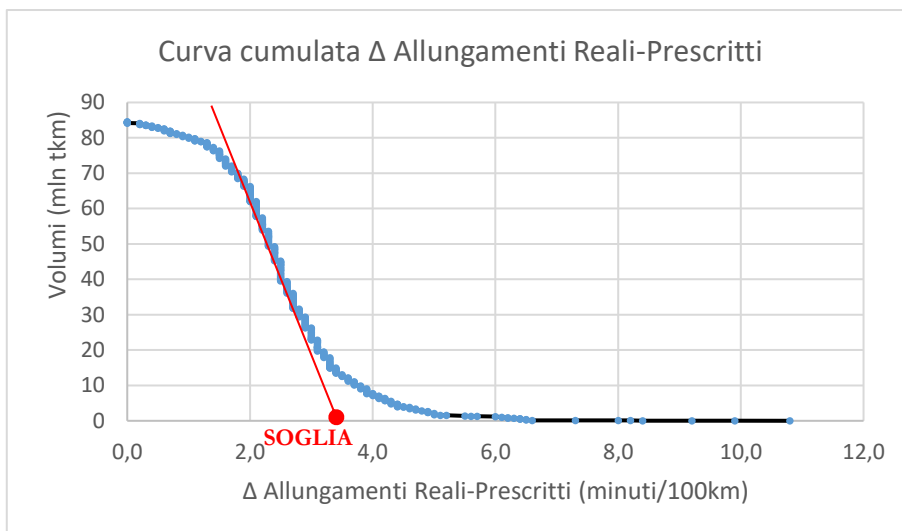
Figura 22 - Curva cumulata allungamenti reali-prescritti (PREMIUM - anno 2023)
